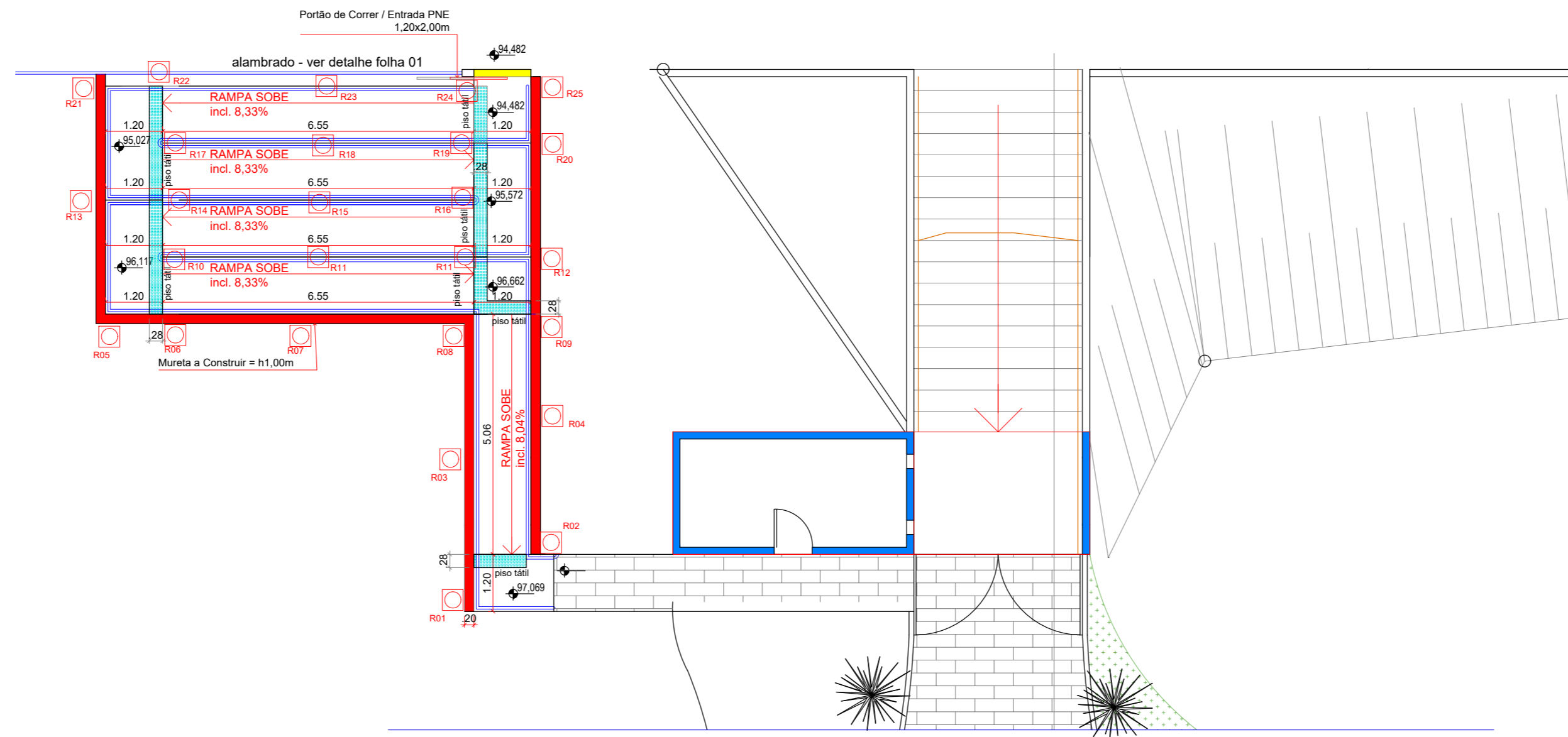
Planta ■ Entrada Principal - esc:1:100
