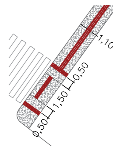
ACESSIBILIDADE - DETALHE 02 S/ Escala
