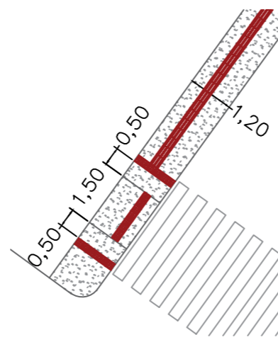
PAVIMENTAÇÃO - DETALHE S/ Escala
