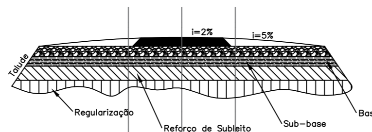
PAVIMENTAÇÃO - DETALHE S/ Escala
