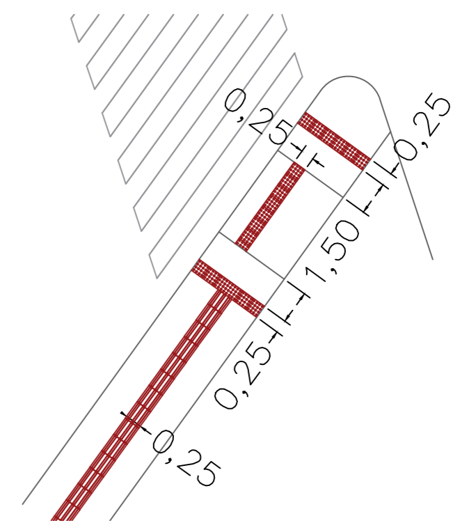
PISO TÁTIL - DIMENSÕES
